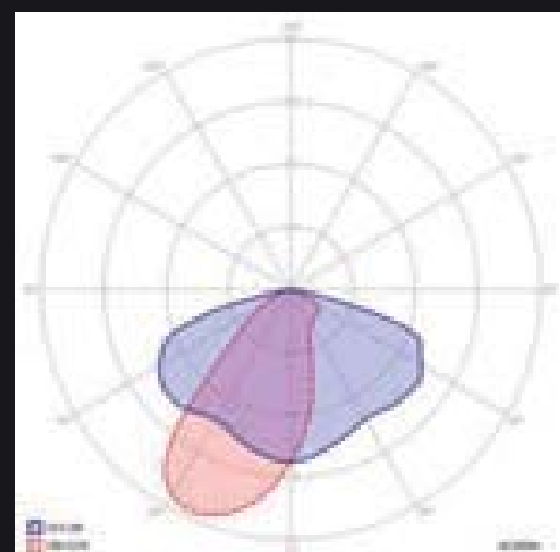
Curva fotometrica
