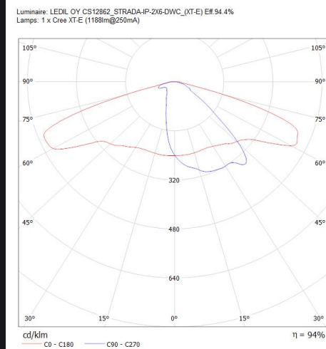
Ottica Ledil 6x2
